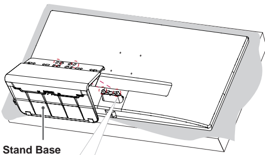
Stand Base
